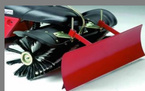
Нож-отвал
